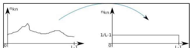
HISTOGRAM EQUALISATION
